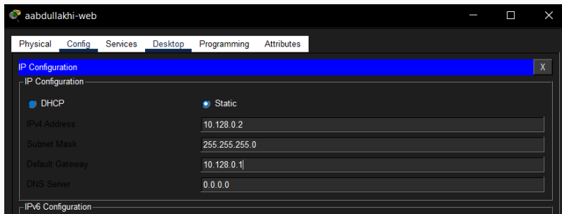
Рис. 7: Web-сервер
